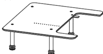
Přídavný stůlek J11862
