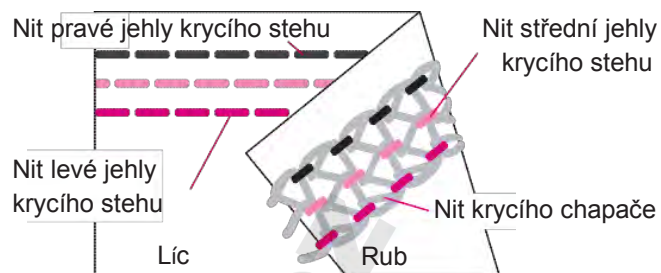
(4) Třínitný krycí steh
